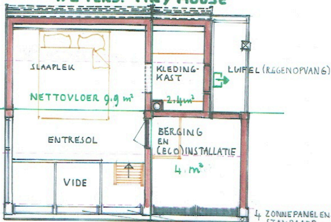
VERDIEPING (ENTRESOL)
