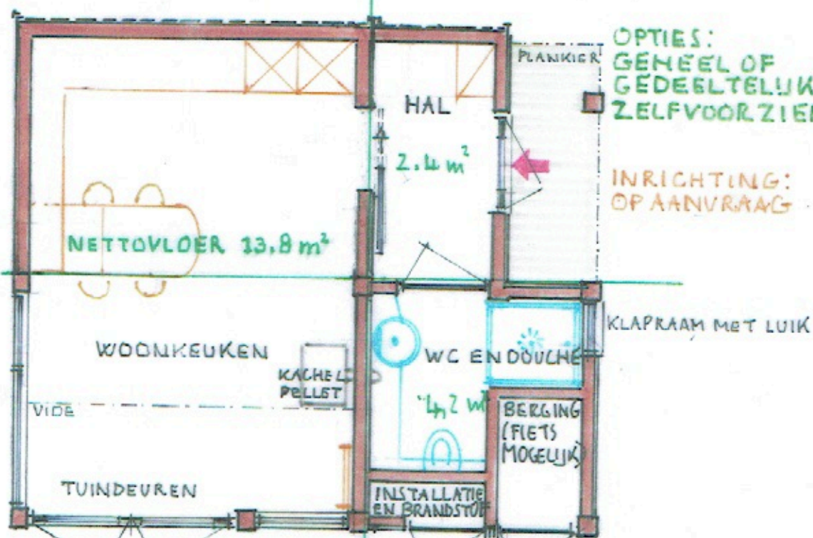
BEGANE GROND
